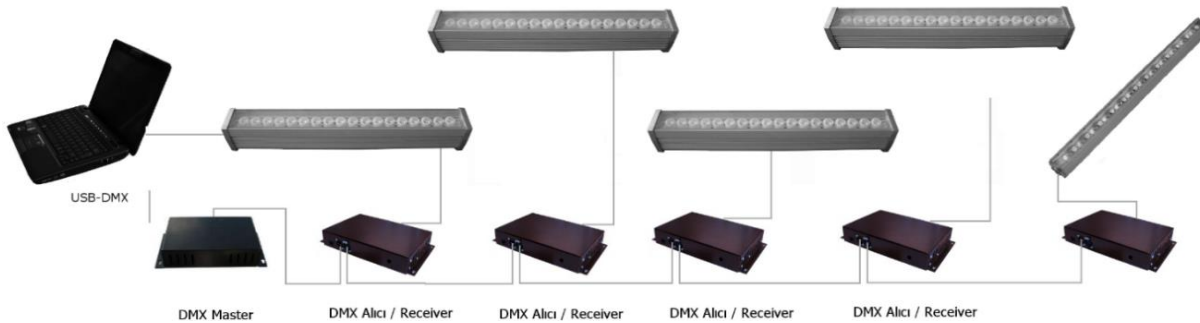
DMX Bağlantı Şeması / DMX Connection Diagram
